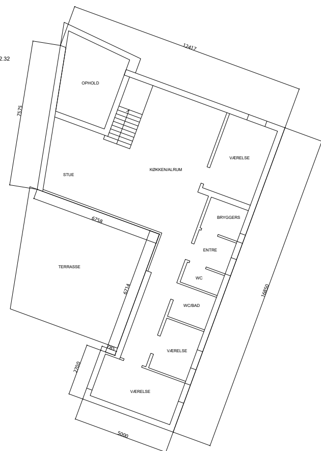
PRINCIP FOR PLAN BRUTTOETAGEAREAL = 130 m 2
